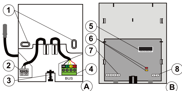
Figure 1 : A – Base; B – Partie frontale du logement contenant l'électronique; 1 – Orifices de montage; 2 – Bornier du capteur externe JB-TS-PT1000; 3 – Vis de verrouillage du capot; 4 – Bornier du bus; 5 – Numéro de série; 6 – Inutilisé; 7 – Goupilles de connexion du bornier du BUS; 8 – Goupilles de connexion du bornier du capteur externe
