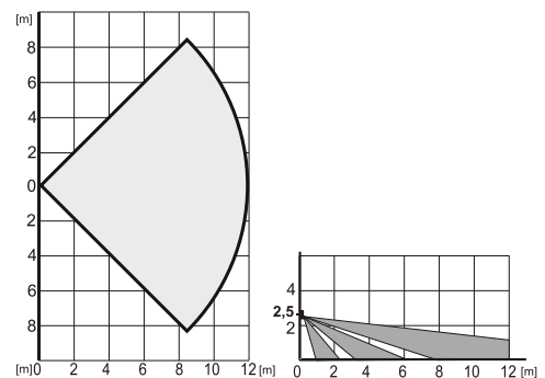
Afbeelding 3: Deze detectiekenmerken gelden voor standaard PIR-immuniteit.
