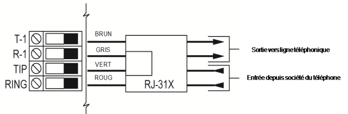
Figure 1-6 Câblage de ligne téléphonique
